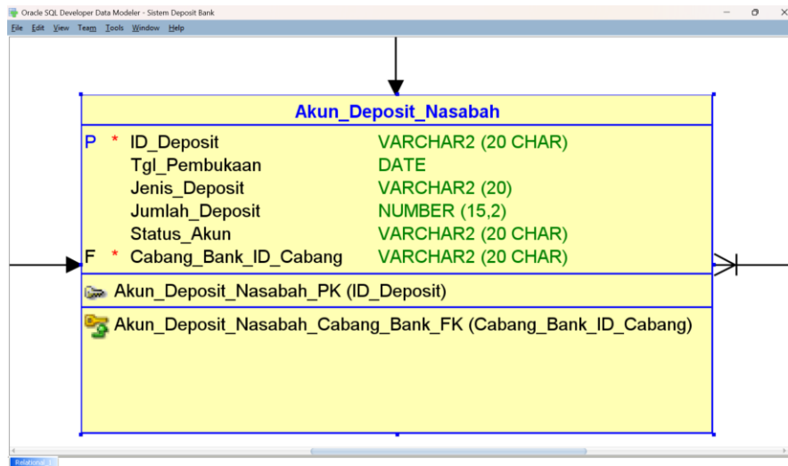
Gambar 2 Atribut dan Keterangan pada Entitas Akun_Deposit_Nasabah
